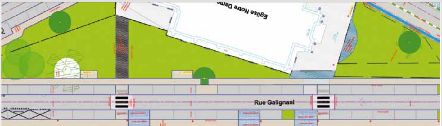
> Rue Galignani Travaux de voirie (reprise des tapis, des bordures, des trottoirs et de l'éclairage public). À noter la création de stationnements des deux côtés de la voirie. De mi-janvier à mai 2018 (4 mois de travaux)
